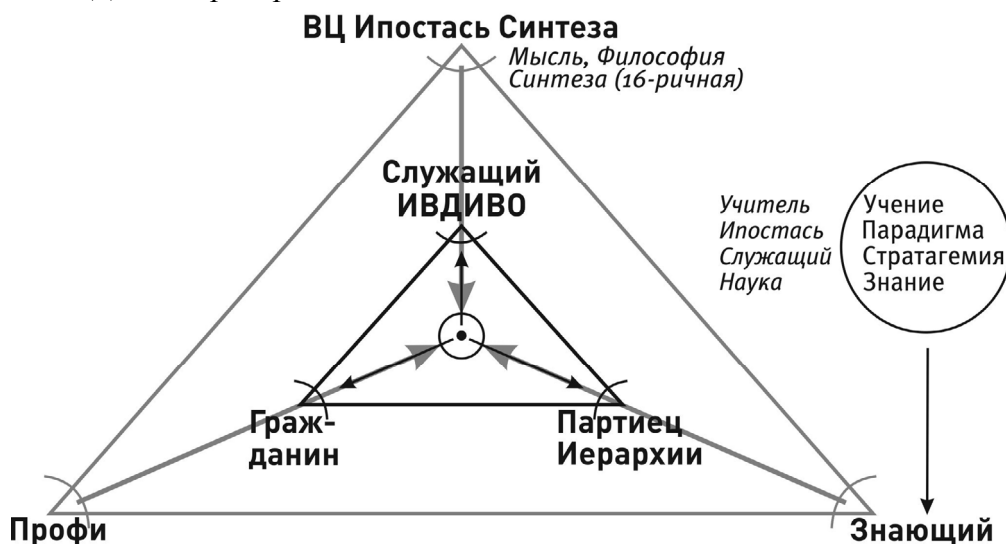
Рисунок 5. Два тетраэдра.
